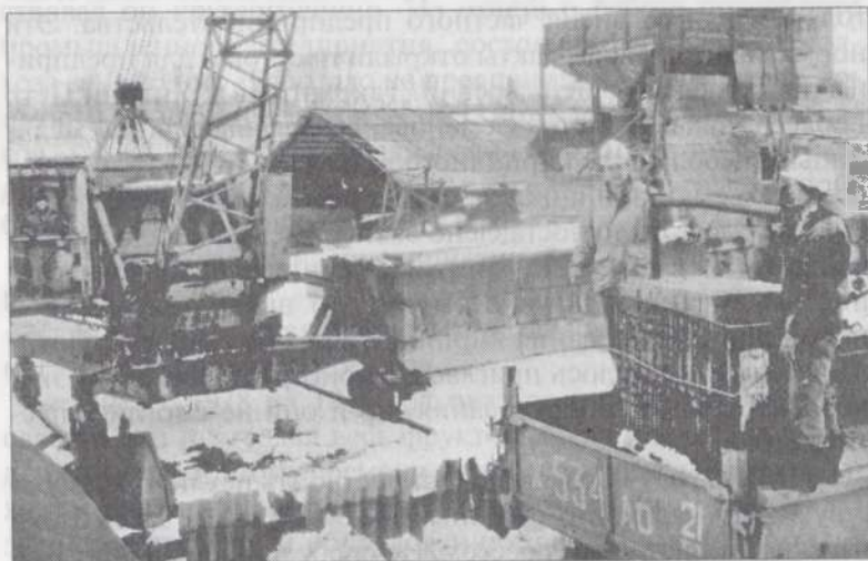
Погрузка керамзито-бетонных блоков на заводе П.А.Гордеева.
