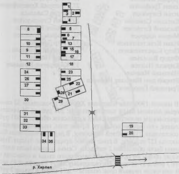
План деревни Кивьялы Норусовской волости Ядринского уезда Казанской губернии снят и составлен страховым агентом Ядринской уездной земской управы Антоном Терентьевым. В мае 1882 года утвержден губернатором Казанской губернии.
