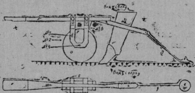
1-мёш ўкерчёк. Върлях тарăна каясран чараканни. а—каток, б—поводок, в—кронштейн, г—сошник, д—сăнчър, е—ункă.
