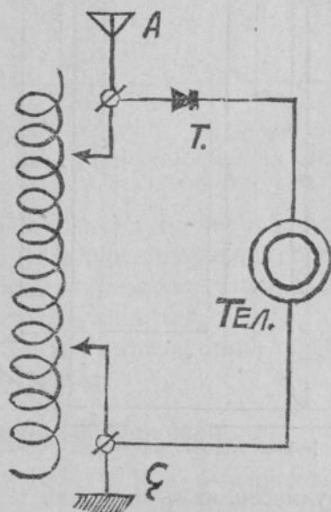
17-мӳш ӳӳррӳк. Прийнмӳнӳк схеми (планӳ).
