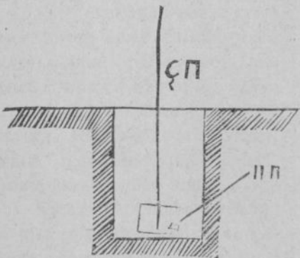
16 мёш ўкерёк. Саçемлени. „çп“ — çёре анакан провйт. „пп“ — пйхйр листа.
