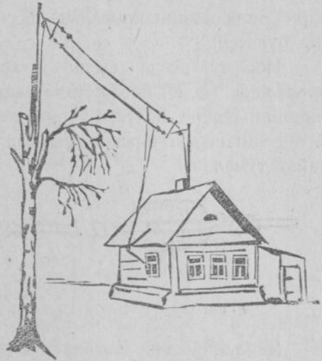
6-мĕш ўкерçĕк. Икĕ провăлкăллă «Г» саспалли йевĕрлĕ антеннă. Маўтисем: пĕри пўрт çинçе, тепри йавăç çинçе.
