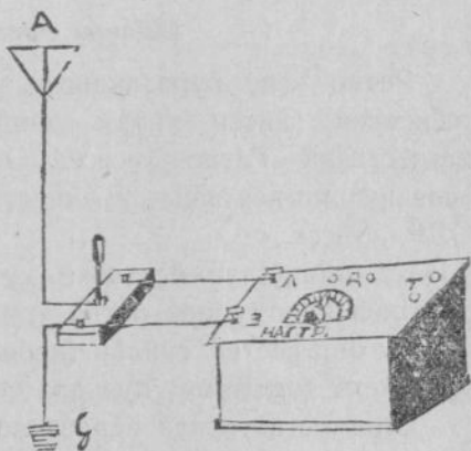
23-мѣш ўкерѹѹк. Хапрăкра тунă приём- нёке лартниие кѣартни.
