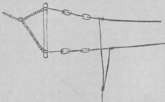
9-мѣш ўкерҗѣк. Антенна пѣр вѣсѣ. Сылтѣмра уславса тѣракав провѣт—приёмник патне анакан провѣт. Сулахайра патака кантѣрапа мѣнле ҫыхнине кѣтартнѣ. Варривҗе исоҗаттѣрсем.
