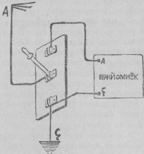
15-мёш ўкерёк. Приёмнёке кросовой перекўбузаттёл сўмне лартни.
