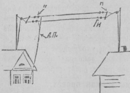
7-мĕш ўкерçĕк. Антеннă маўтисем пеккĕшине те пўртсем сине лартнă. „И“—изоляторсем, „П“—патак, „А П“—анакан провăт.
