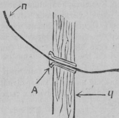
13-мёш ўкерзёк. Приёмнёк патне анакач провāта пўрте кўртни. „П“ провāт, „А“ кёпсе, „Ч“ зўрефе рамё.
