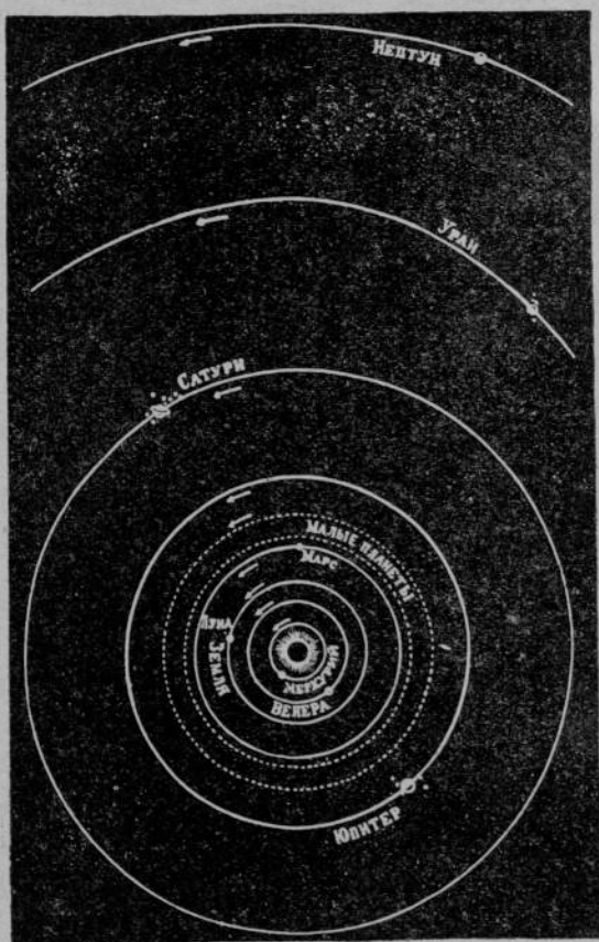
50-мёш карт. Хёвел тавра ҫавәрәнакан планетсем.
