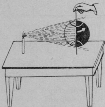
8-мёш карт. Ҷёр хёвел умёнҶе хай йёри-тавра Ҷавараннипе кунпа каҶ мёнле пулса пынине катартаҶ.
