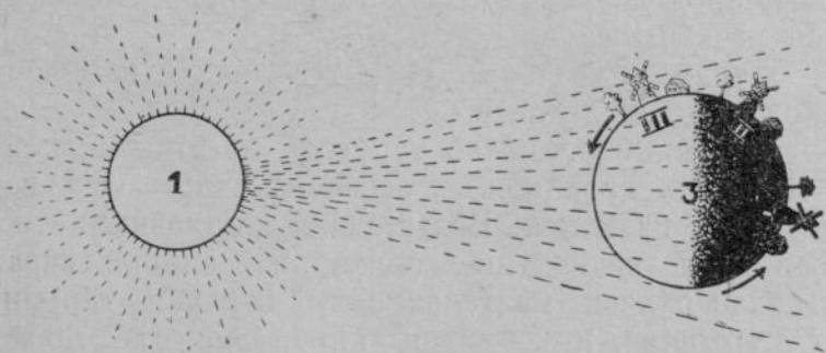
1-мөш картинә. 1 — хёвел, 3 — сёр. Стрелкәна сёр хай тавра хәш йенелле саврәннине кәртәнә.
