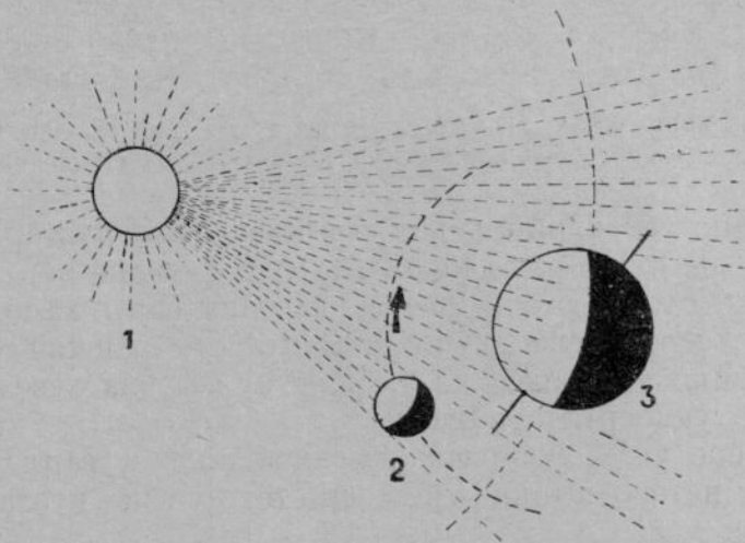
25-мәш карт. 1—хәвел; 2—уйәх; 3—сёр. Уйәх хәвелпе сёр хушшинелле савәранса пыраәт.
